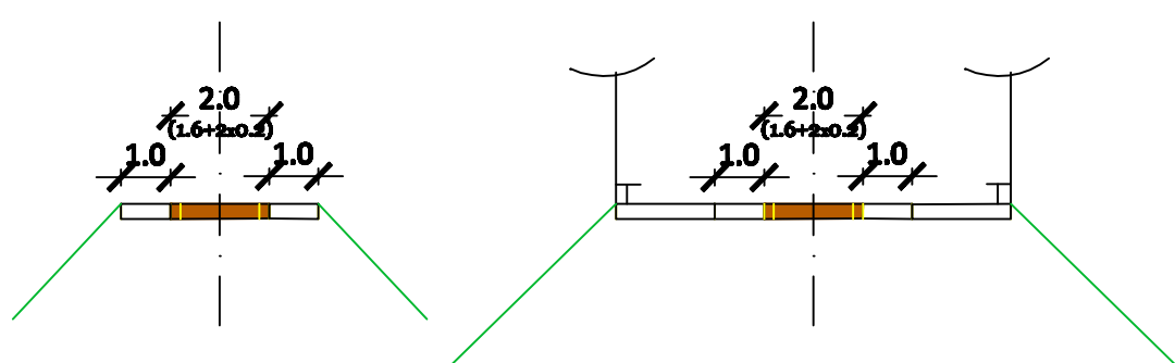
ПОПРЕЧНИ ПРОФИЛ 3-3
