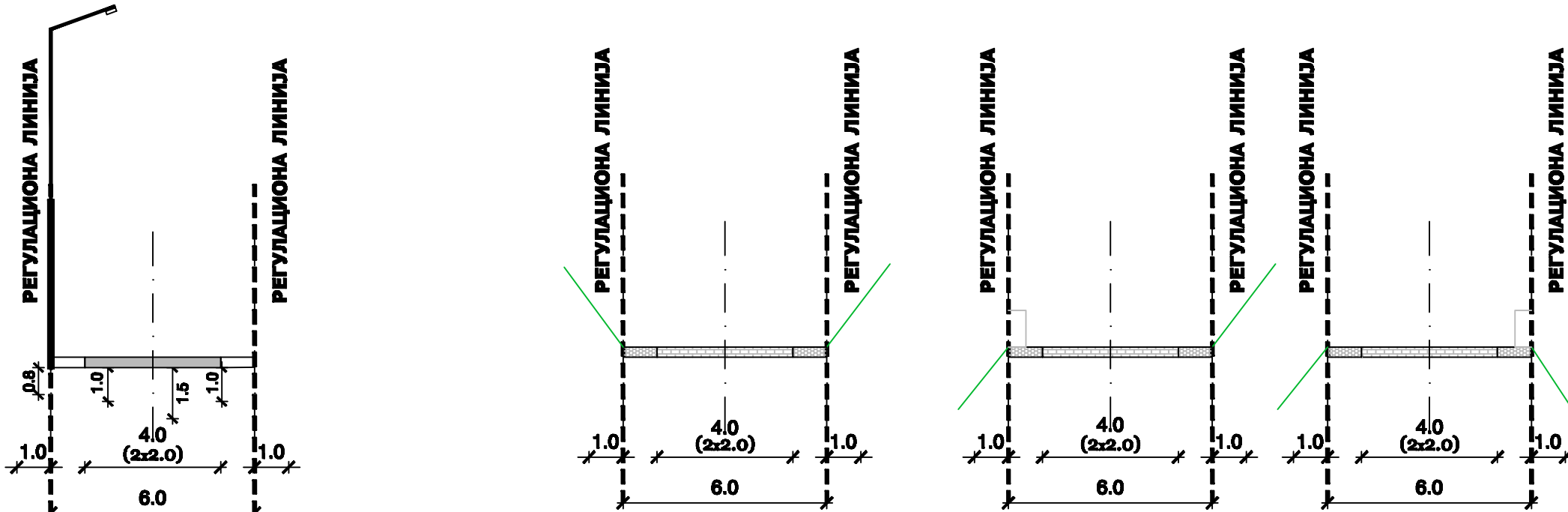
ПОПРЕЧНИ ПРОФИЛ 2-2
